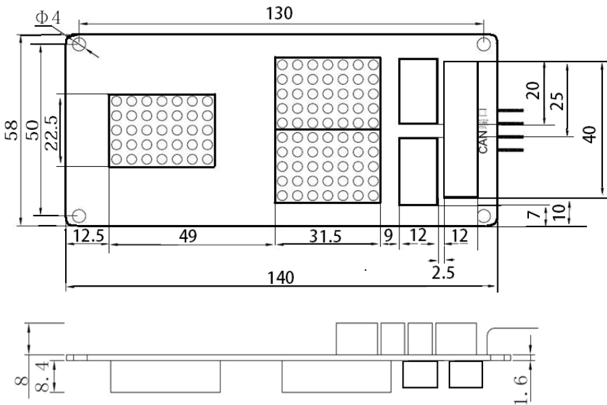
图 1 DC-03A 安装尺寸图
