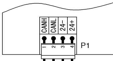
图2 呼梯显示板通讯总线 P1 电气接口（端子型号：VH-4）
