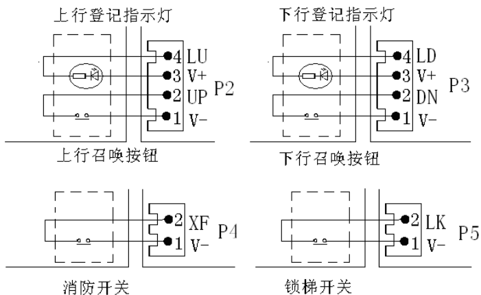
图 4 呼梯显示板通讯总线电气连接
