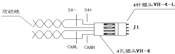
图3 呼梯显示板与电源和通讯总线的连接方法
